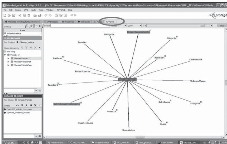
Figura 4 – A interface do plug-in TGVizTab, exibindo o conceito <wheeled vehicle> no centro do grafo.
