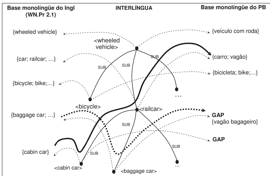
Figura 5 – Os alinhamentos léxico-conceituais na base de dados REBECA.
